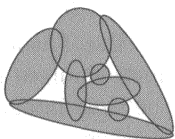
pseudodisks
